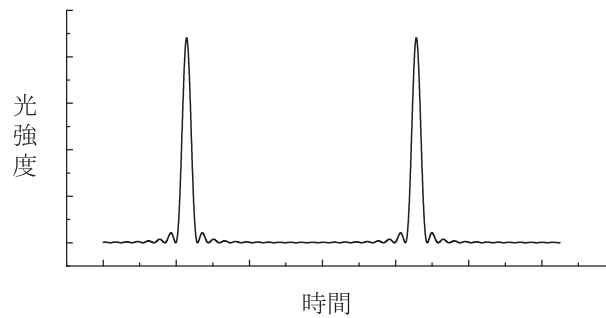
図 2.16: モード数が 21 の場合の、モード同期レーザーの出力光強度
