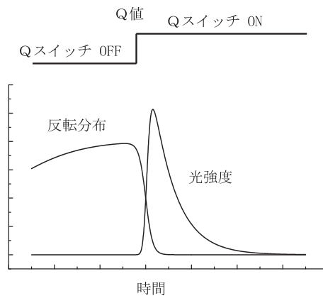
図 2.15: Qスイッチレーザーにおける時間発展
