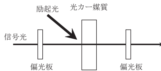
図 6.9: 光カーシャッター
