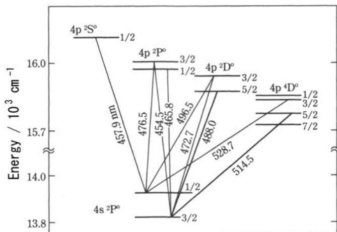
図 3.5: アルゴンイオン ( \text{Ar}^+ ) のエネルギー図
