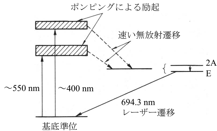
図 3.2: ルビーレーザーのエネルギー図
